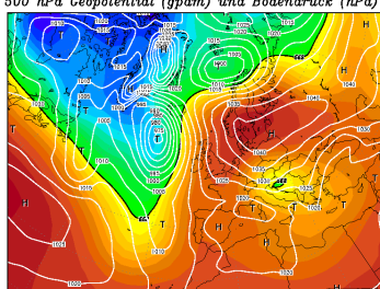
07NOV2003 00Z 500 hPa Geopotential (gpm) und Bodendruck (hPa)
