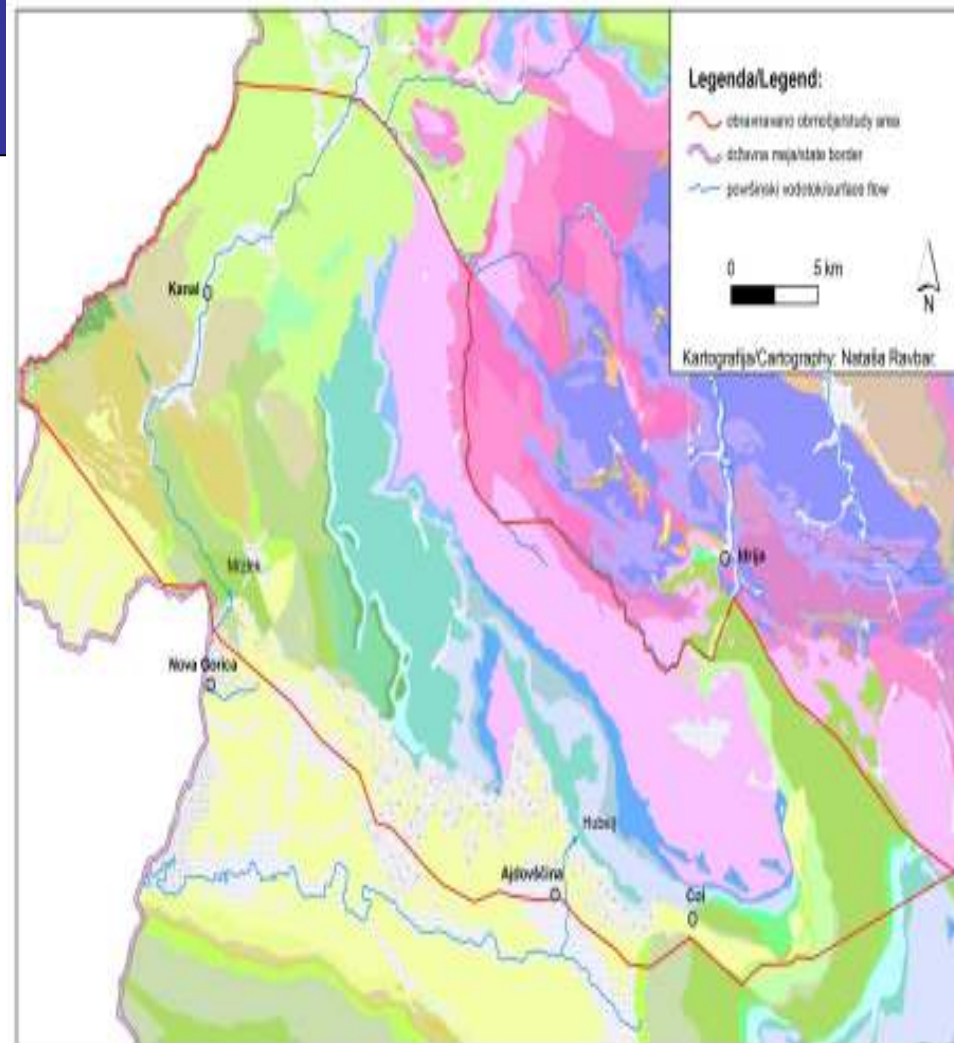
Slika 2: Geološka karta Trnovsko-Banjške planote z omejenim območjem, ki je vključeno v kraški hidrogeološki model GEP Vir: IZRK ZRC SAZU
